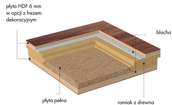
KONSTRUKCJA SKRZYDŁA DIAMENT
