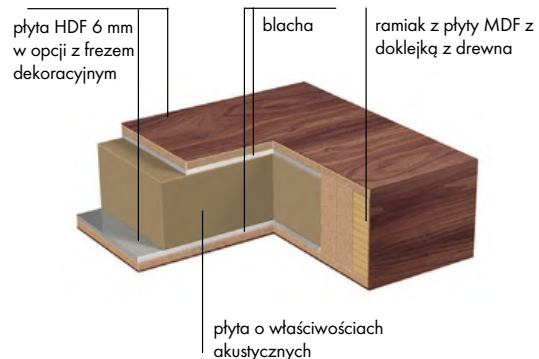
KONSTRUKCJA SKRZYDŁA TOWER STRONG
